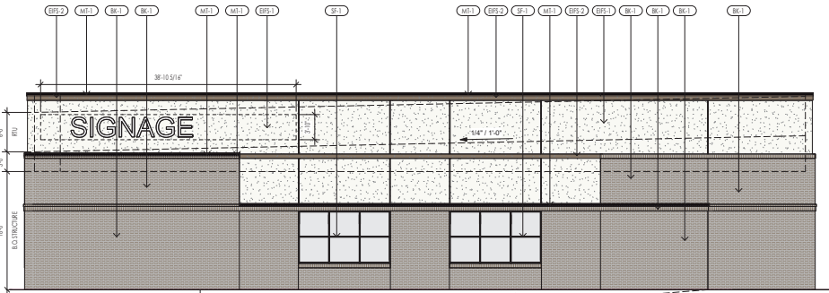
ELEVATION 4 SCALE: 1/8" = 1'-0"
