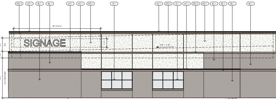
ELEVATION 4 SCALE: 1/8" = 1'-0"
