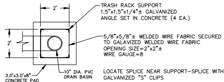
B-B RISER PIPE PLAN N.T.S.
