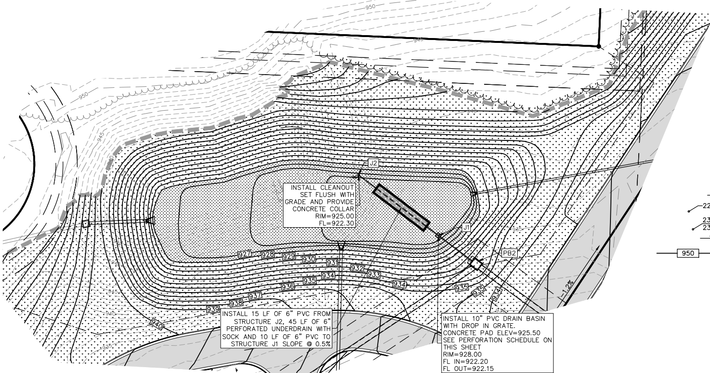
B-B RISER PIPE PLAN N.T.S.
