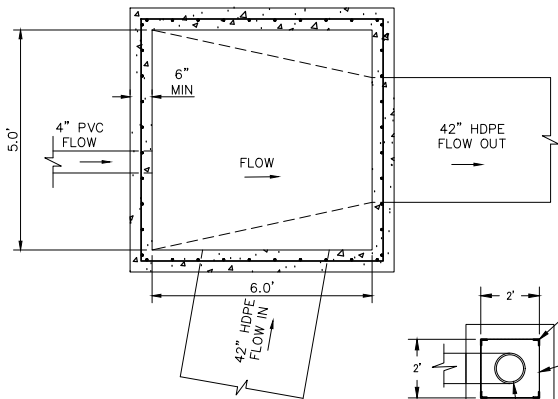
B-B RISER PIPE PLAN N.T.S.
