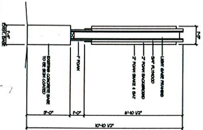
SIGN SECTION SCALE: 1/2" = 1'-0"
